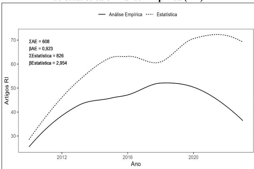
Gráfico 3 – Expansão da Incidência ( \alpha ) de estatística e Análise Empírica (AE)
