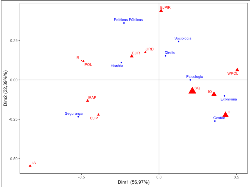
Gráfico 5 – Análise de Correspondência (CA) dos campos mais influentes
