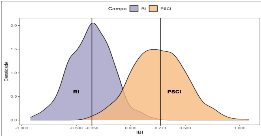
Gráfico 2 - Distribuição de IBI e distância de Hellinger
